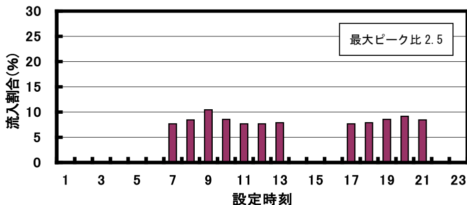
図 2-7 試験用原水流入パターン (501 人槽以上)
