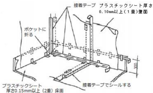
図1 床の隔離養生例
