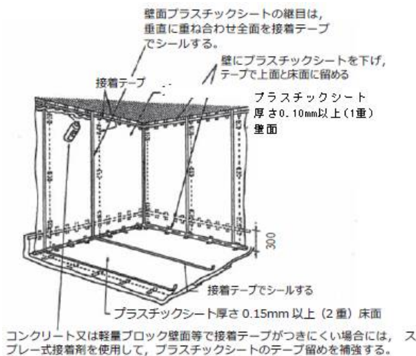
図2 壁部の隔離養生例
